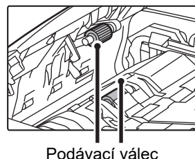
Podávací válec
