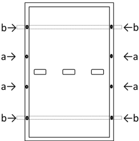
Bild A3: Positionen der Montagelöcher für Schraubmontage
