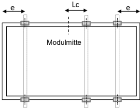
Bild A1: Klemmenposition an langer Rahmenseite
