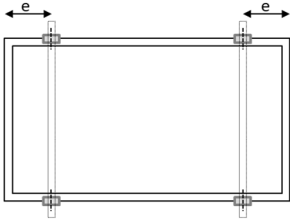
Bild A2: Klemmenposition an langer Rahmenseite
