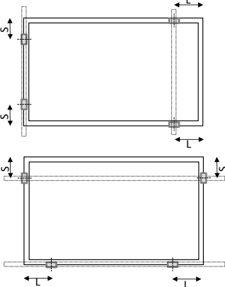
Fig. B: Posición de las sujeciones en los marcos corto y los marcos largos
