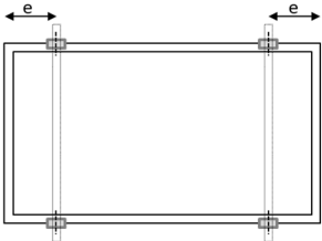
Schéma A2: Position de fixation par clip sur le côté long des cadres
