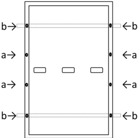
Schéma A3: Emplacement des trous de boulon
