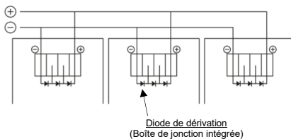
Schéma 2. Parallèle pour plus de courant
