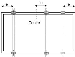
Schéma A1: Position de fixation par clip sur le côté long des cadres
