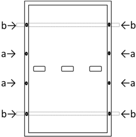
Fig. A3. Ubicación de los orificios para pernos
