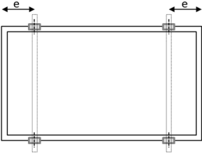
Fig. A2. Posición de las sujeciones en el marco largo
